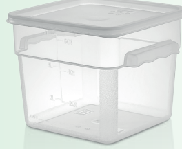
GSPP-6 5.7 Lt - 192 Oz Square Container Kare Saklama Kabı 6 pcs /ctn Şeffaf / Clear 242 x 232 x 191 mm
